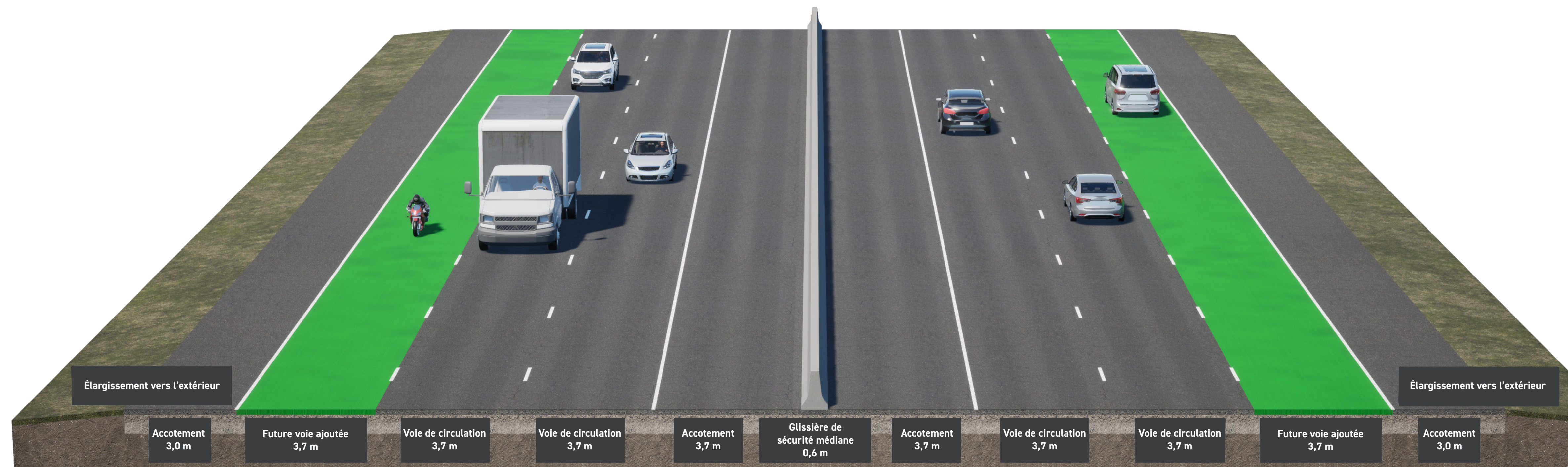
RPGC 101 en direction sud RPGC 101 en direction nord Section transversale de la RPGC 101 typique à six voies (futures voies ajoutées vers l'extérieur)
