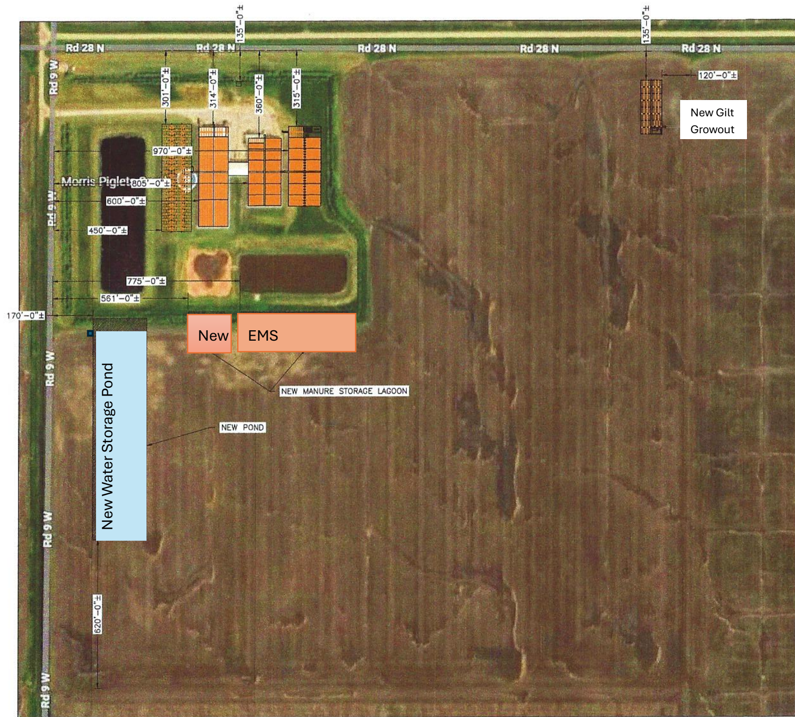
Morris Piglets Site Layout
